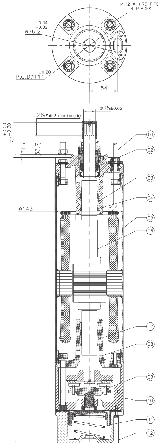
MOTOR-A
